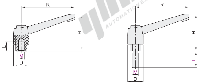
内螺纹型 E-HAF32
