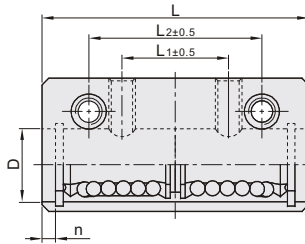
双衬型 E-LMY01
