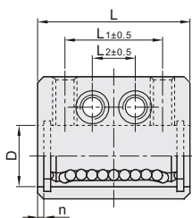
单衬型 E-LMX01
