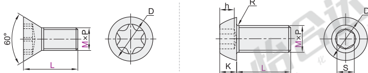
梅花槽型 TAU51
