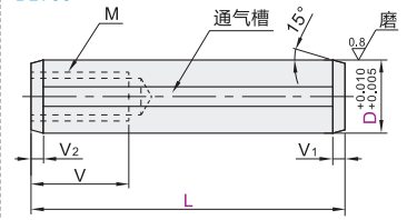
带通气槽型·公差 +0.010 / +0.005 经济型
