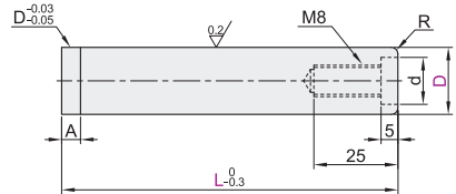
压入型·固定挡块 OFJ13
