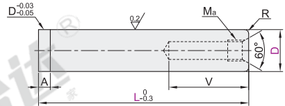
压入型·固定挡块 OFJ13
