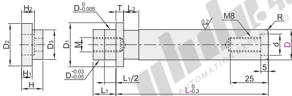
装卸型·固定挡块 OFJ03
