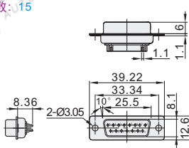
插针头 ZIS10 P数: 15
