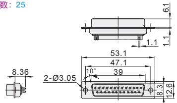
插针头 ZIS10 P数: 25
