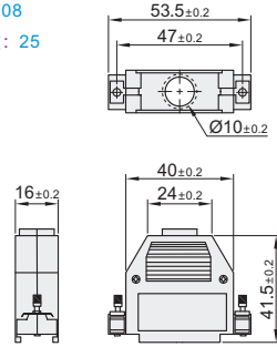
插孔头 ZIS09 P数: 25
