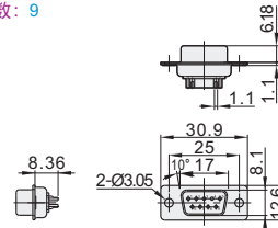
插针头 ZIS10 P数: 9
