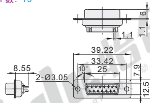
插孔头 ZIS09 P数: 15
