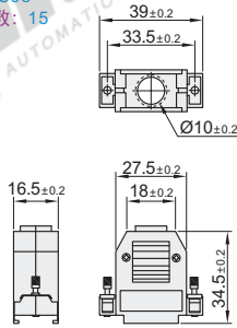
插孔头 ZIS09 P数: 15
