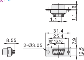
插孔头 ZIS09 P数: 9
