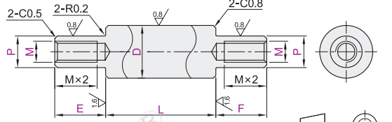
两端内螺纹型 MCF01~86
