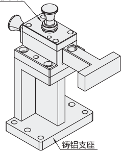
滑移机构
