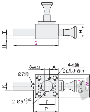
直杆型 PGB27 W=40
