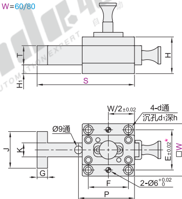
滑移机构
