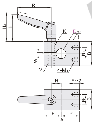
螺孔平行标准型 REC01/02
