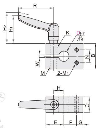
螺孔垂直薄型 REC21/22
