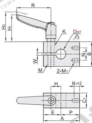
螺孔平行薄型 REC11/12
