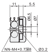
截面AA
