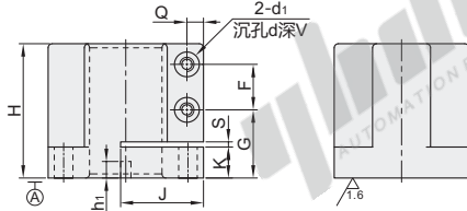
底座 ZCD01
