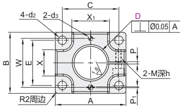
锁块 ZCD11
