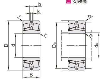
安装图
