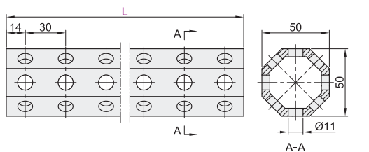
铝型材中空八角管 BWL02
