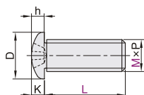
十字槽盘头螺钉
