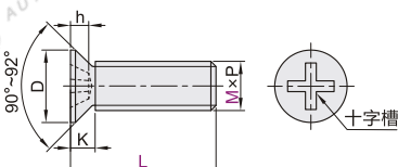
十字槽沉头螺钉
