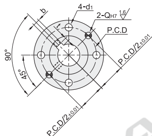
圆法兰型 GAU21/22
