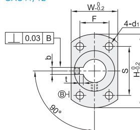
对边法兰型 GAU11/12
