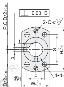
对边法兰型 GAU31/32
