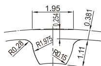
标准齿形
