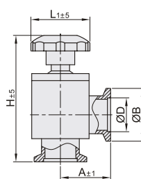
XLQ03 (铝)
