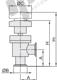
BLQ50 (SUS304)
