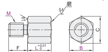
B尺寸指定·F尺寸固定型 YML91/92/93/94/95
