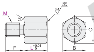
B-F尺寸固定型 YML71/72/73/74/75
