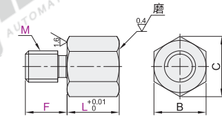
B尺寸固定·F尺寸指定型 YML81/82/83/84/85
