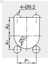
安装开孔尺寸
