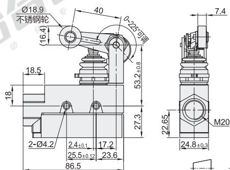
H: 带密封圈V铁架滚轮型
