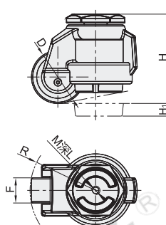
丝杆活动型 J-CXB06
