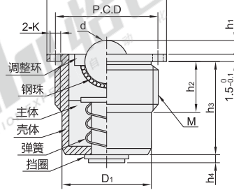
柱塞螺纹型 QDF02
