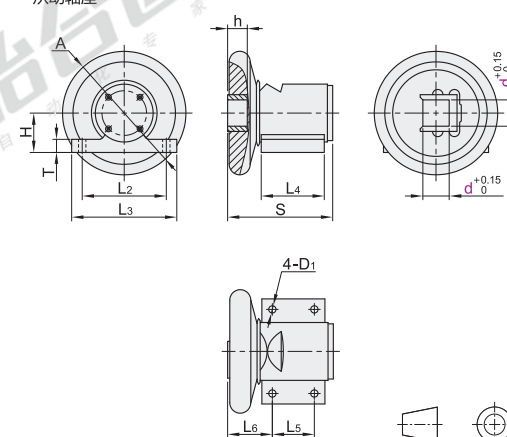
从动轴座
