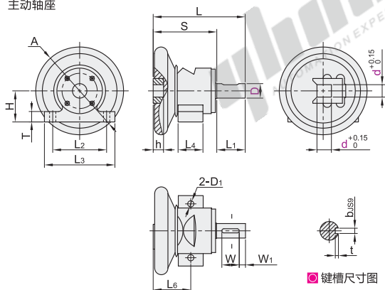
D28/D35
