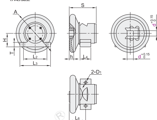
从动轴座
