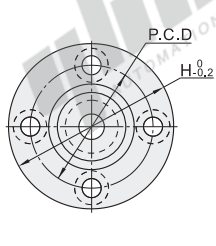
圆法兰 E-BFU31/32/33/34/36
