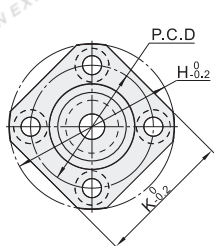
方法兰 E-BFU41/42/43/44/46
