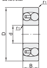
圆柱孔型
