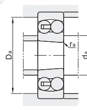
安装图
