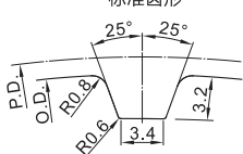
标准齿形
