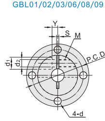
圆法兰型
