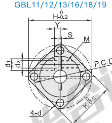
方法兰型
