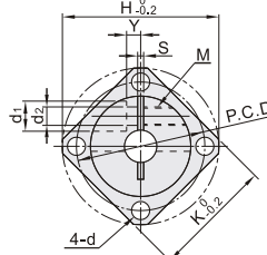
方法兰型
