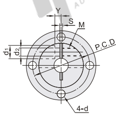
圆法兰型
