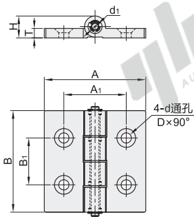
4孔安装
