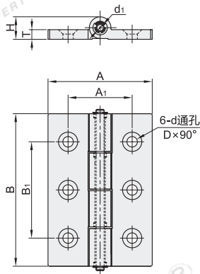
6孔安装
