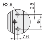
❑ B处放大图
