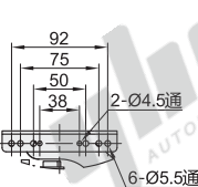
❑ C处放大图
