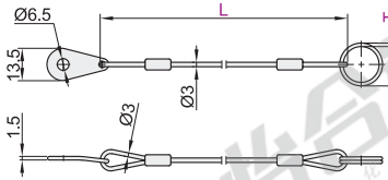
一端环型一端耳型 ZAA43
