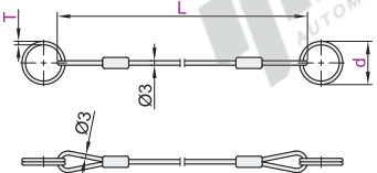
两端环型 ZAA41
