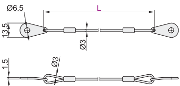
两端耳型 ZAA42
