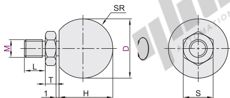
外螺纹型 HAJ91
