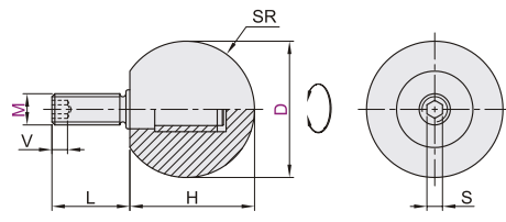
外螺纹内六角孔型 HAJ93
