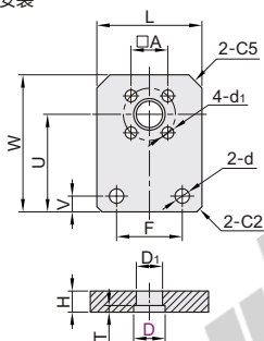
气缸安装形式：螺母安装
