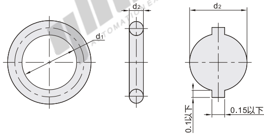
截面放大图
