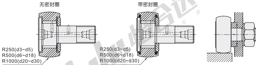
标准型·全滚针球面型 BPF27/28
