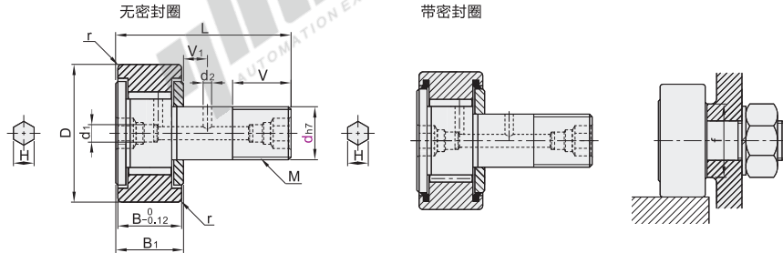
标准型·全滚针圆柱型 BPF07/08
