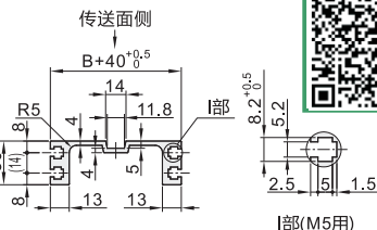
型材截面放大图
