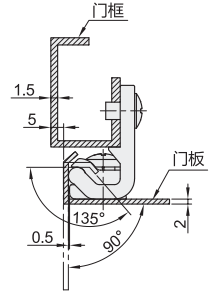
□ HFR34安装示意图
