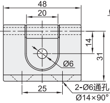
内折型 HFS61
