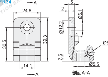
方型 HFR34
