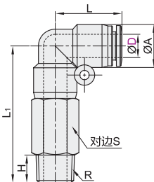
加长弯接头 XZS07
