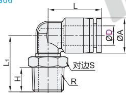
弯接头 XZS06
