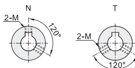
安装方式 (键槽+螺孔)
