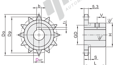
链轮 VLY01/02
