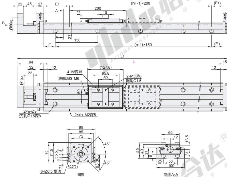
单一滑块螺帽使用之油嘴方向
