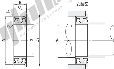
安装图
