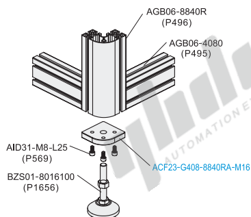
分解图
