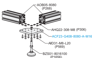
分解图
