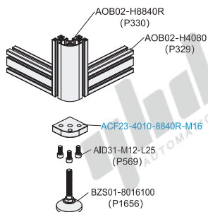
分解图
