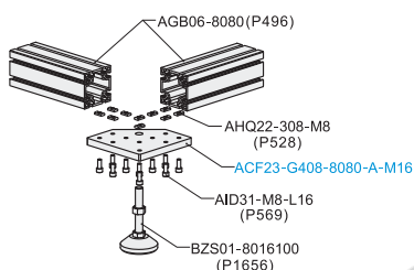
分解图
