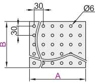
孔加工型 NBS03/13
