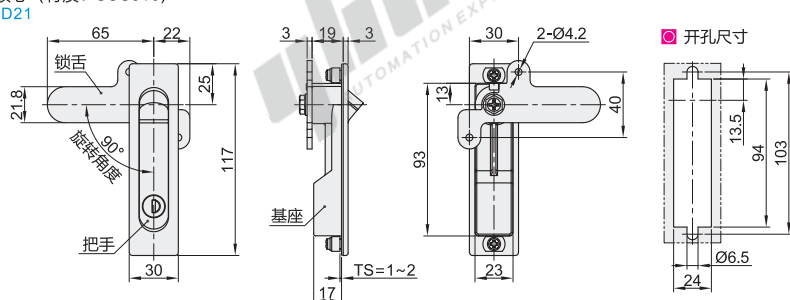
带锁芯 (材质: SUS316)
