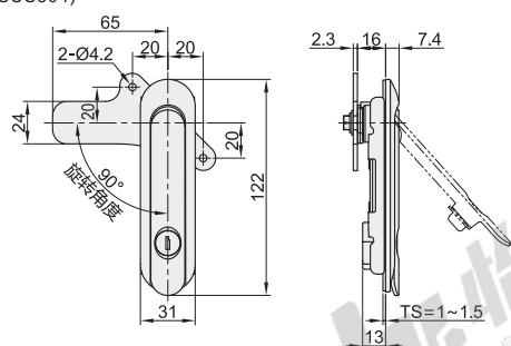
带锁芯 (材质: SUS316)
