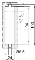
● 开孔尺寸
