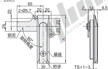
带锁芯 (材质: SUS304)
