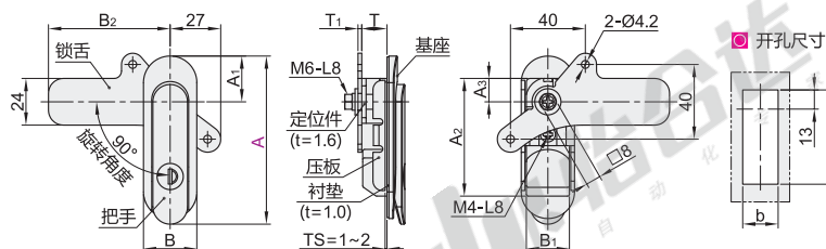
带锁芯 XBD20 (材质: SUS304)
