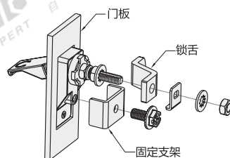
安装分解图
