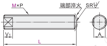
带扳手槽型
