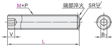
内六角孔型
