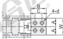
固定端 规格 202/203 204/206 306/408 412
