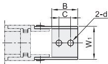
移动端 规格102
