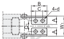
移动端 规格 202/203 204/206 306/408 412
