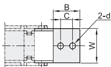
固定端 规格102
