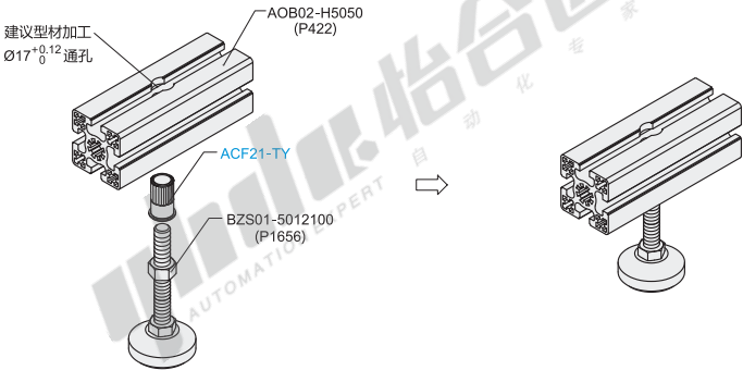
分解图
