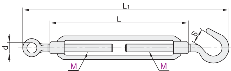
开体式:OC型 TCJ93
