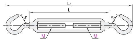
开体式:CC型 TCJ92
