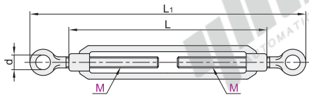
开体式:OO型 TCJ91
