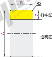
标签展开尺寸图
