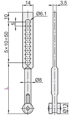
带多孔滚轮连杆 XAV53
